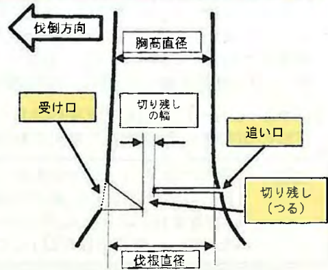
(図1)受け口、追い口等の関係図
